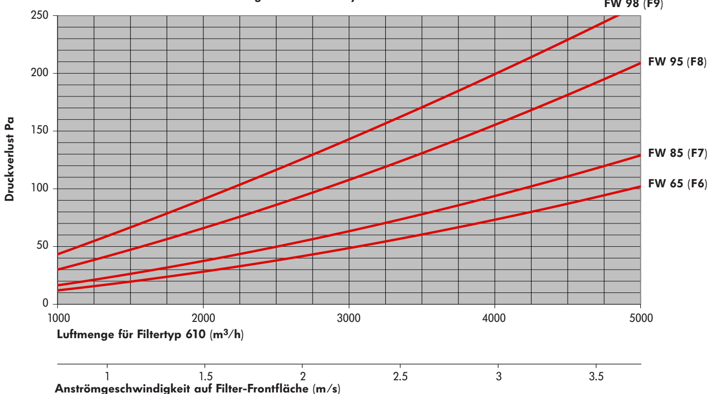
Anfangsdruckverluste SynaWave® Taschenfilter
